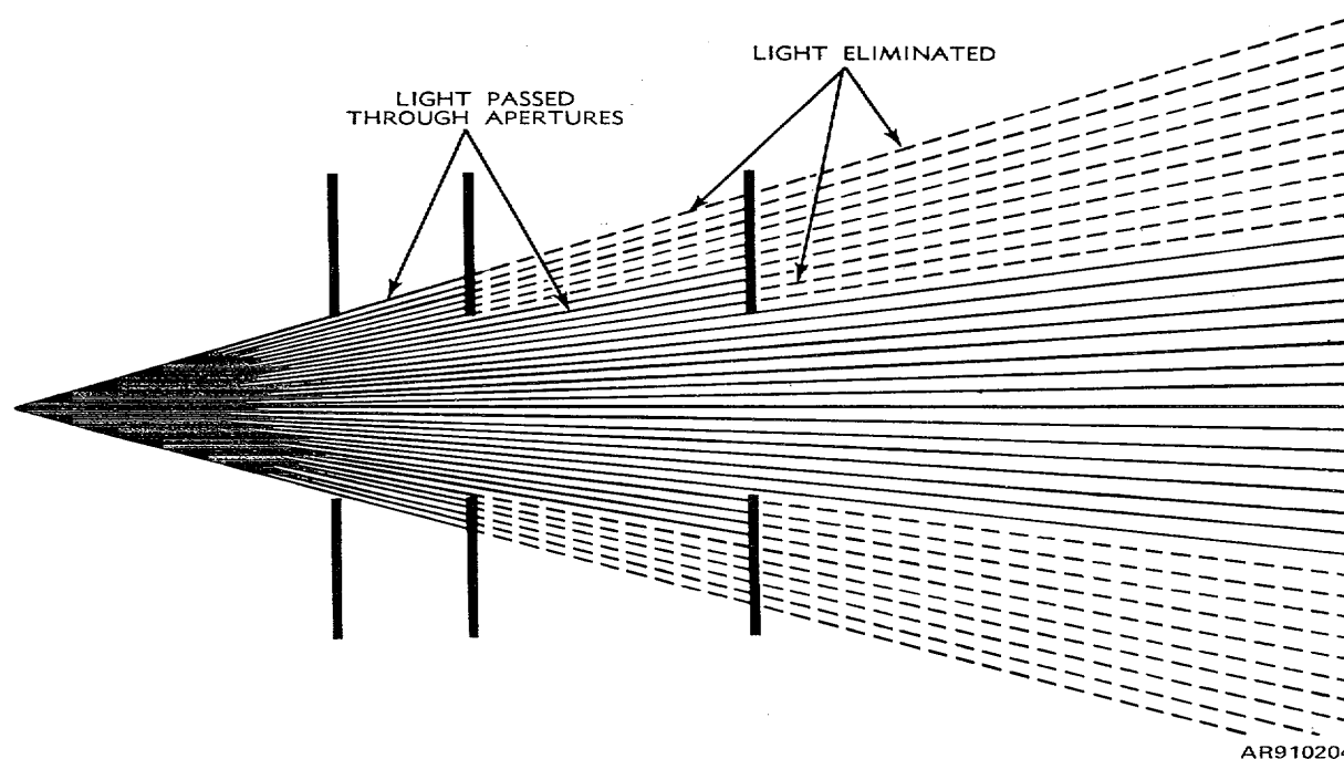
Figure B-4. Apertures.
