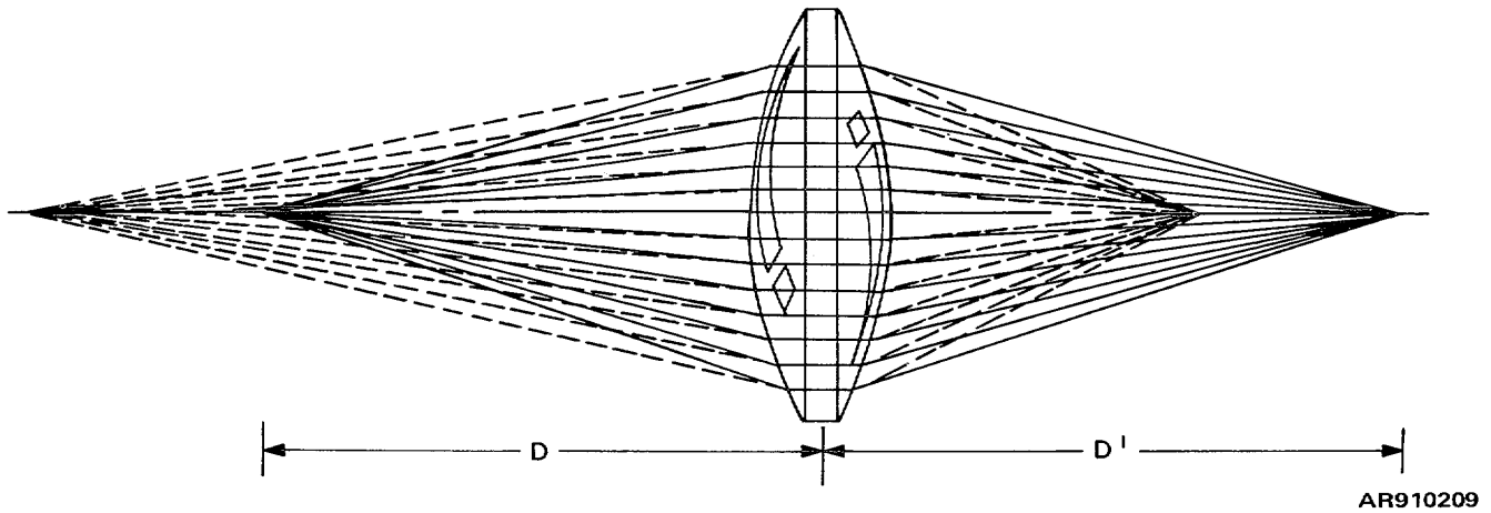
Figure B-9. Conjugate focal points (conjugate foci).
